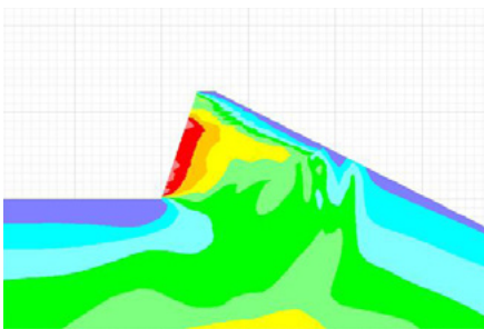
Cálculo dinâmico de impacto de avalanche
