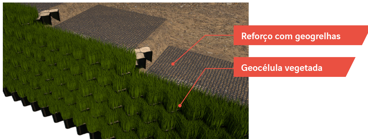
ArmaGreen – paramento com geocélula e geogrelha de reforço
