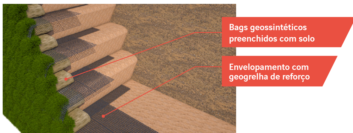
ArmaGreen – paramento com bag geossintéticos envelopado com geogrelha de reforço
